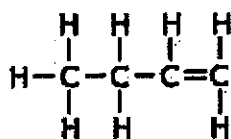
1-butene
