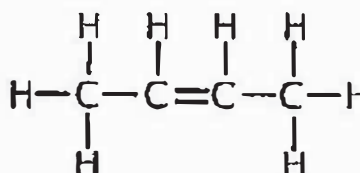
butylene
