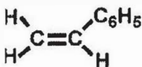
Styrene
