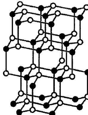
structure Y
